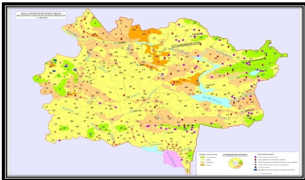
Рис.3 - Зона экологического риска Восточно-казахстанской области
